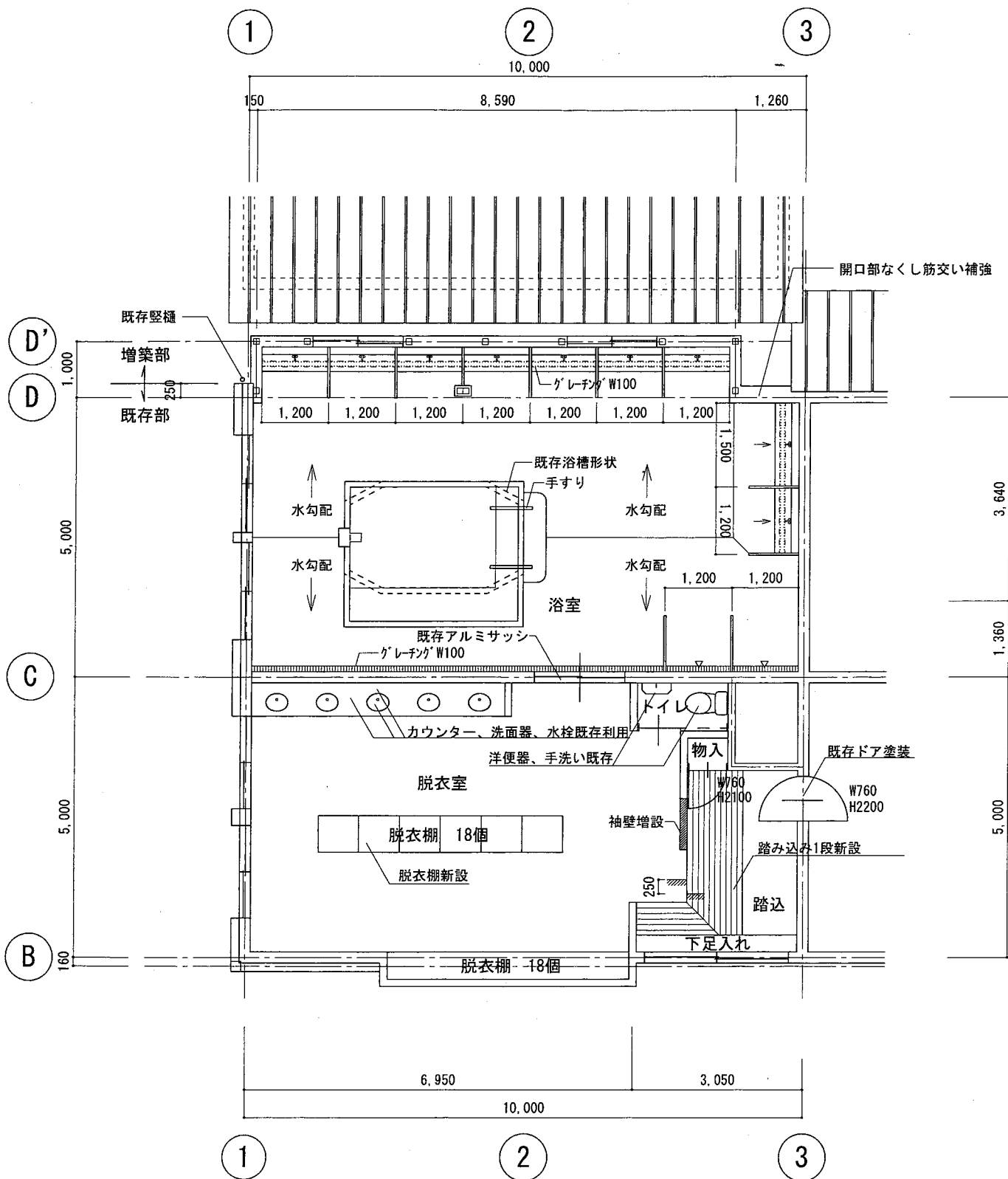
2階平面図
